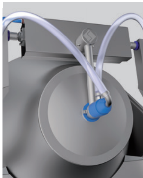
Sistema di carico automatico della salamoia
